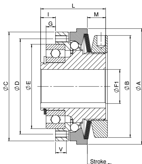
Versione con foro e cava
