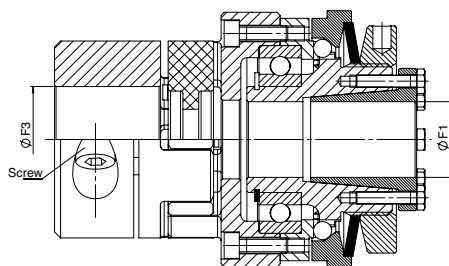
Versione limitatore con calettatore / GESM
