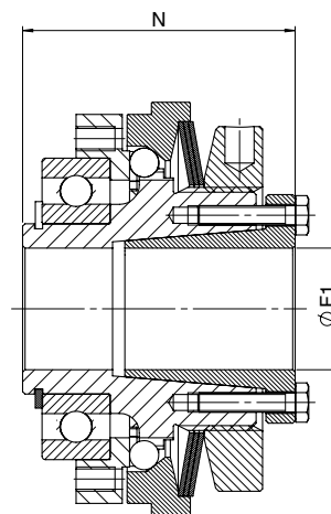
Versione con calettatore
