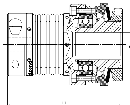
Versione limitatore foro + cava / GSP
