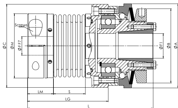
Versione limitatore con calettatore / GSP
